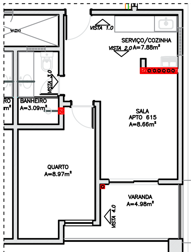
PLANTA APARTAMENTO 615
