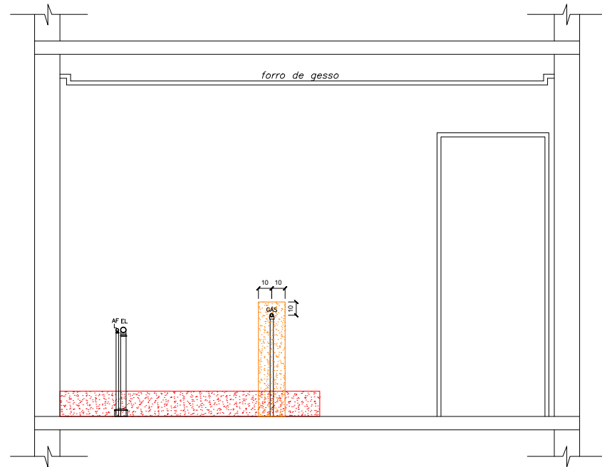
VISTA 1.0 - APARTAMENTO 611
