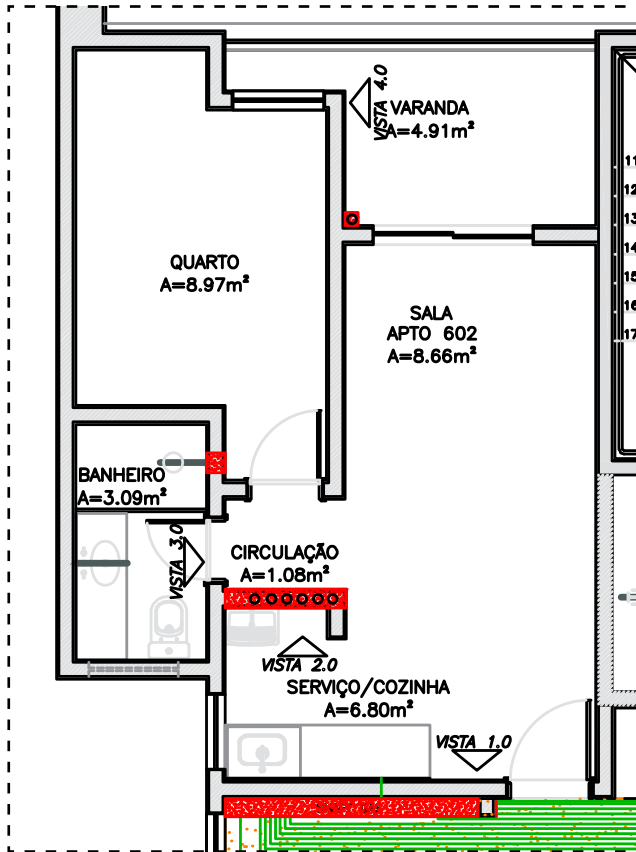
PLANTA APARTAMENTO 602
