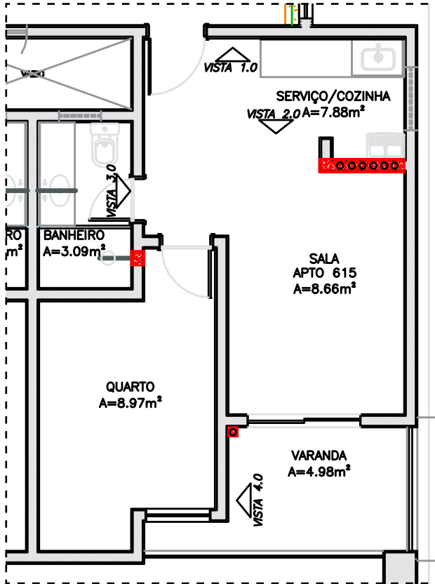
PLANTA APARTAMENTO 615
