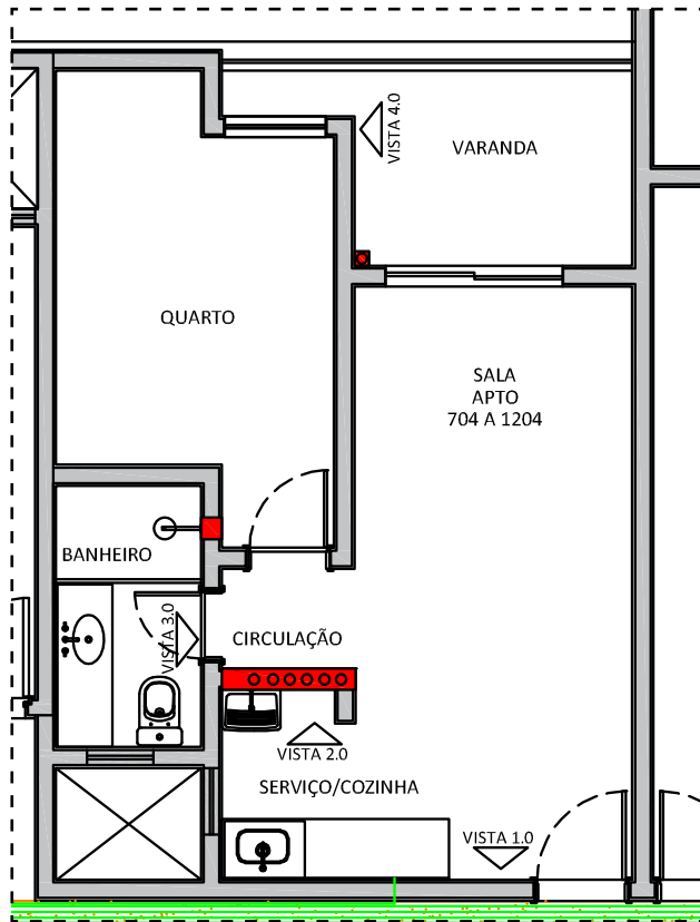
PLANTA APARTAMENTO 704 A 1204
