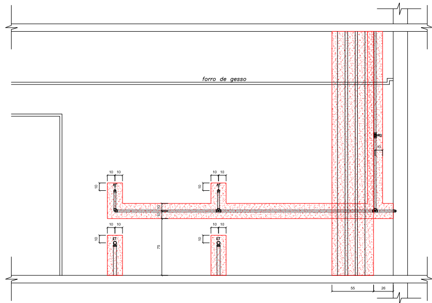
VISTA 3.0 - LAVANDERIA
