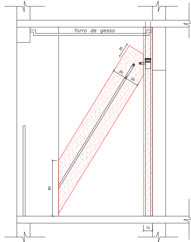
VISTA 4.0 - APARTAMENTO 606
