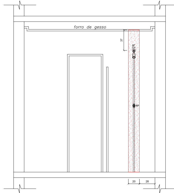
VISTA 3.0 - APARTAMENTO 606
