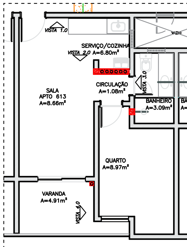
PLANTA APARTAMENTO 613
