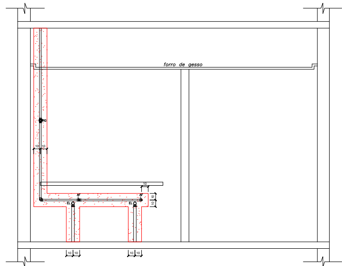
VISTA 2.0 - WC MASCULINO
