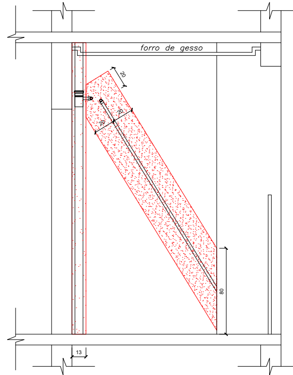
VISTA 4.0 - APARTAMENTO 701 A 1201
