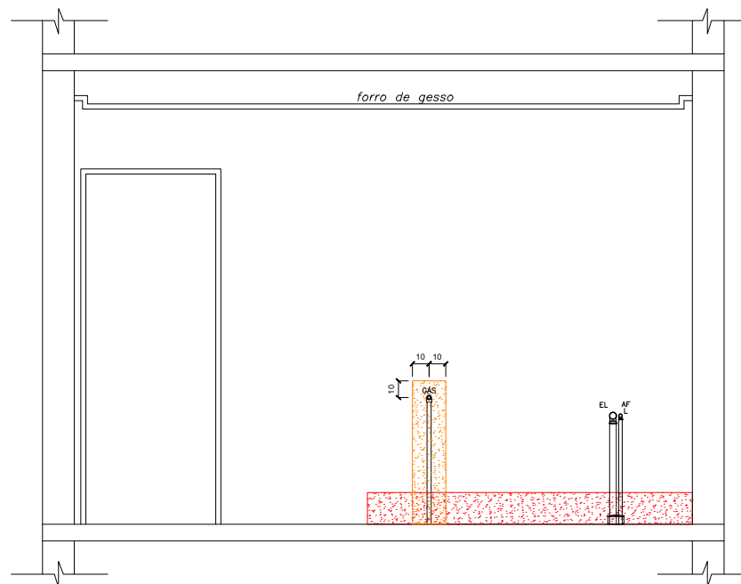
VISTA 1.0 - APARTAMENTO 605
