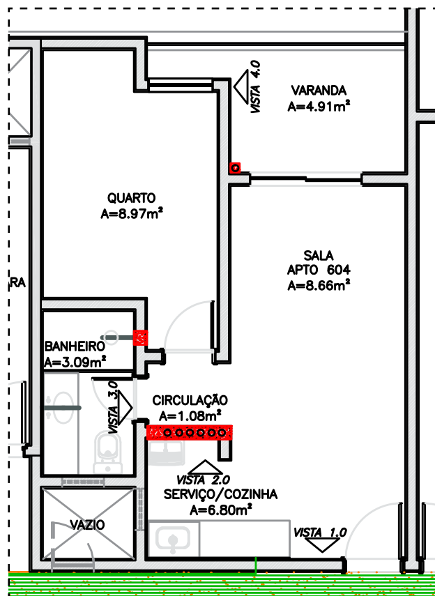
PLANTA APARTAMENTO 604
