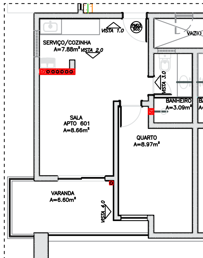
PLANTA APARTAMENTO 601
