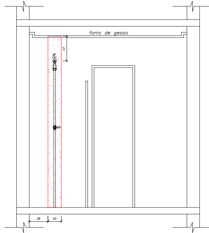
VISTA 3.0 - APARTAMENTO 612
