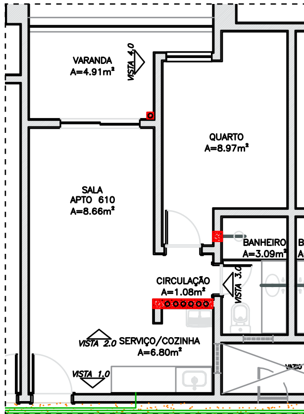
PLANTA APARTAMENTO 610
