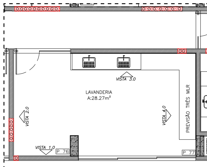
PLANTA LAVANDERIA
