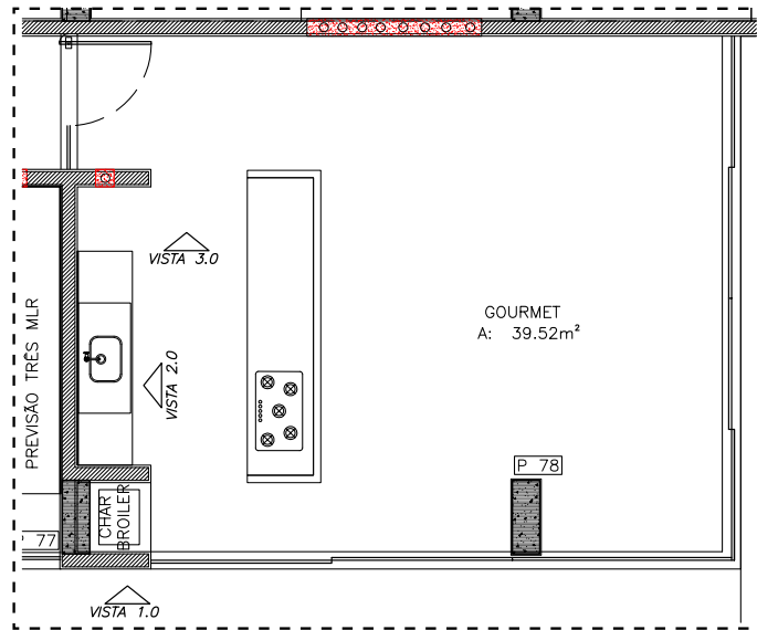
PLANTA GOURMET
