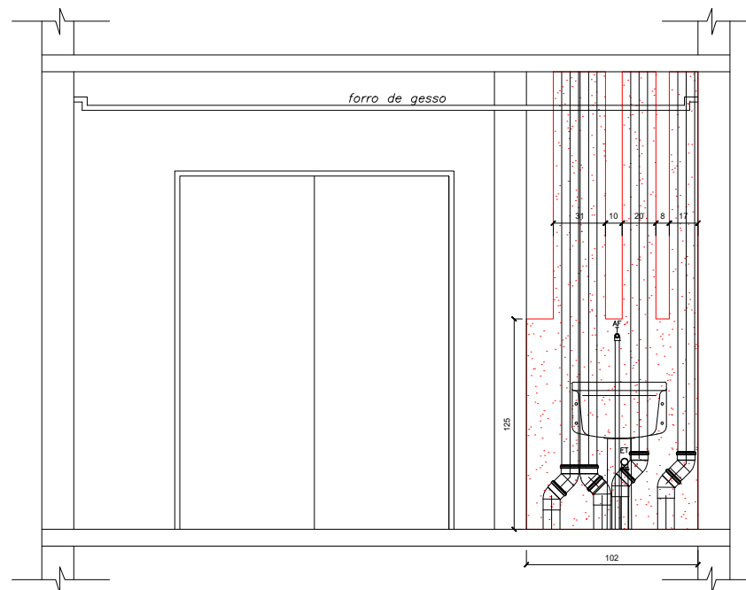
VISTA 2.0 - APARTAMENTO 603
