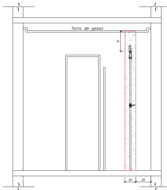
VISTA 3.0 - APARTAMENTO 611
