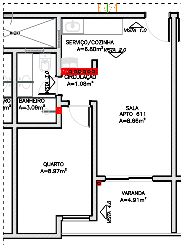
PLANTA APARTAMENTO 611
