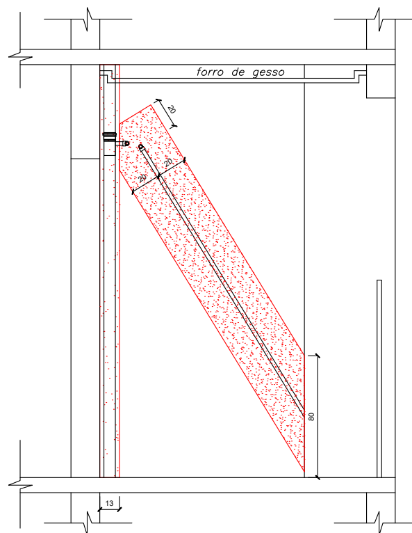
VISTA 4.0 - APARTAMENTO 604
