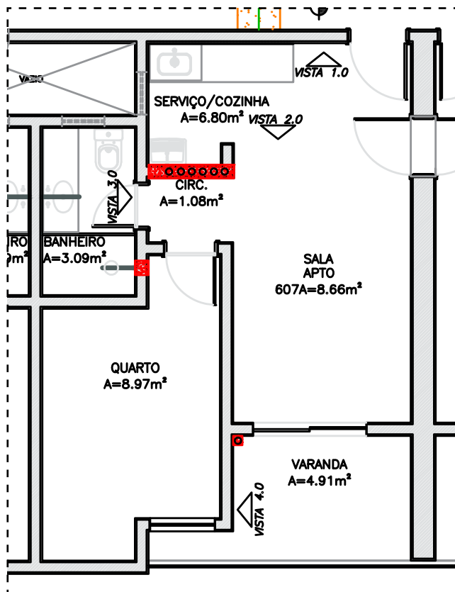
PLANTA APARTAMENTO 607
