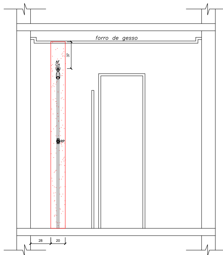
VISTA 3.0 - APARTAMENTO 605
