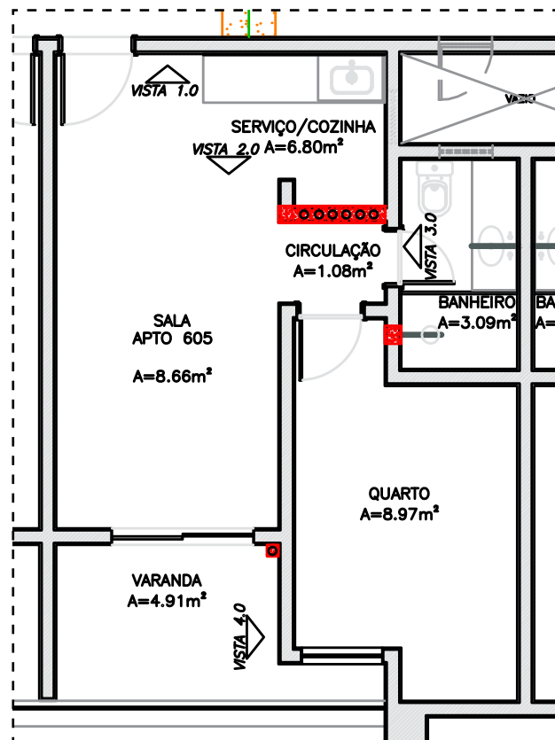
PLANTA APARTAMENTO 605
