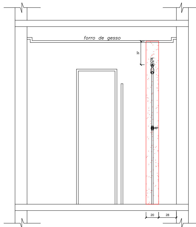
VISTA 3.0 - APARTAMENTO 610
