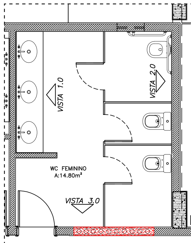
PLANTA WC FEMININO
