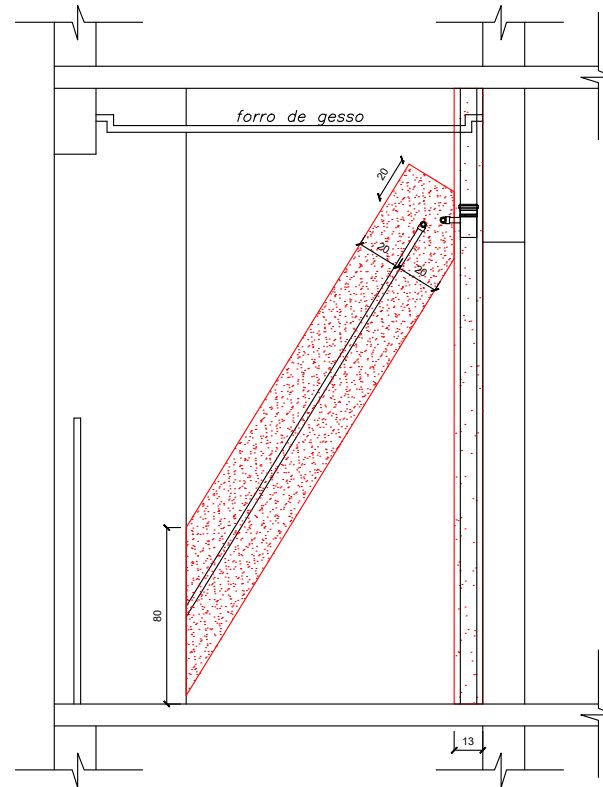
VISTA 4.0 - APARTAMENTO 610
