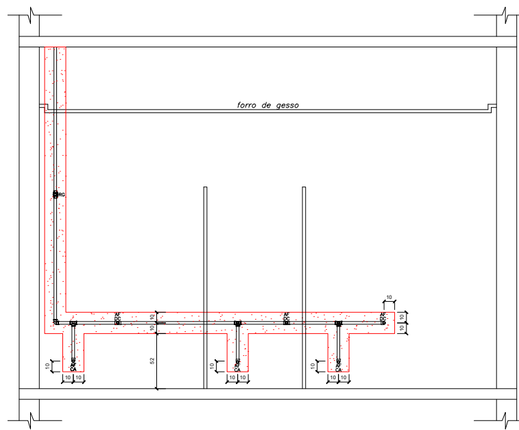
VISTA 2.0 - WC FEMININO
