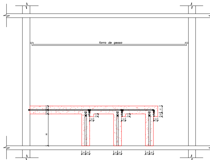
VISTA 4.0 - LAVANDERIA
