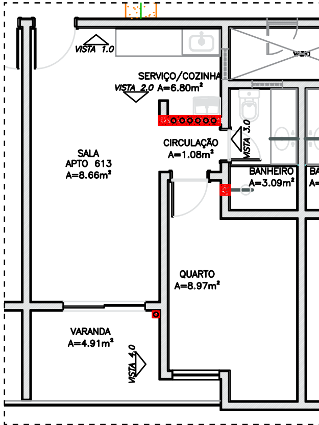
PLANTA APARTAMENTO 613
