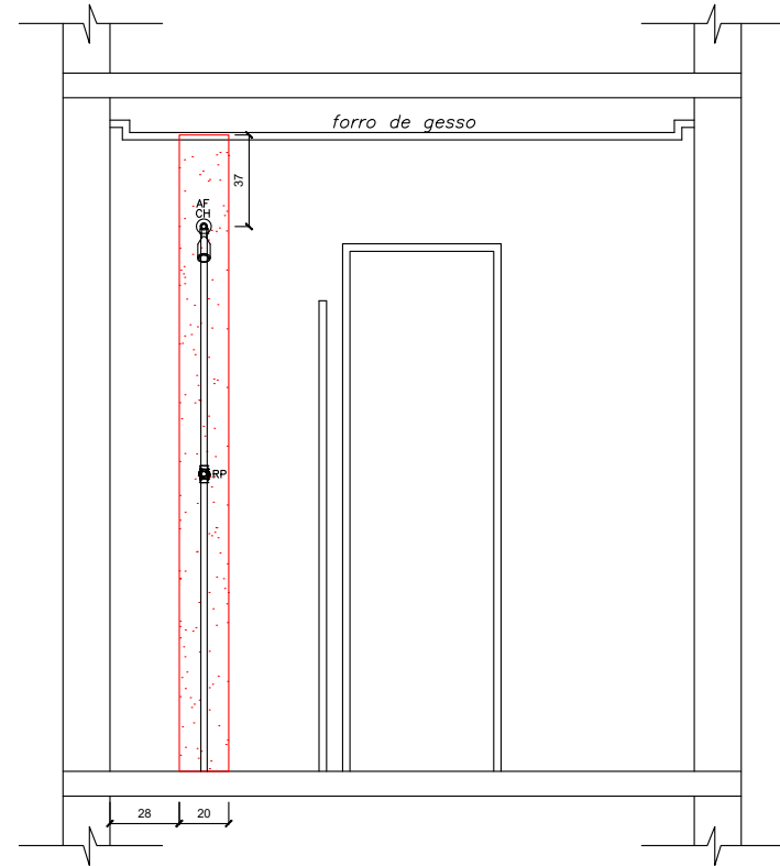
VISTA 3.0 - APARTAMENTO 702 A 1202
