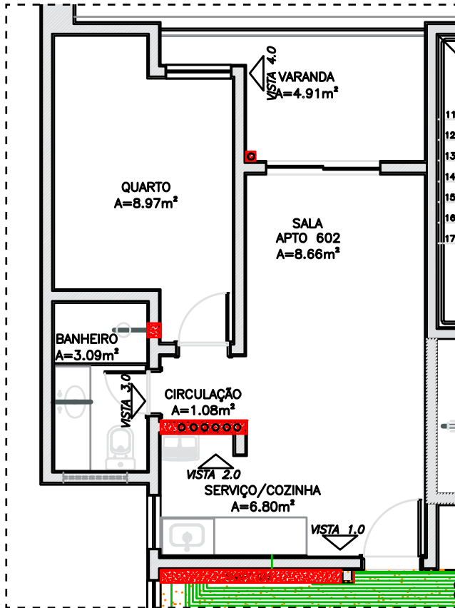
PLANTA APARTAMENTO 602
