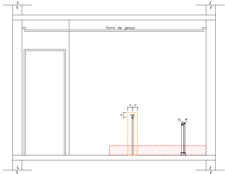
VISTA 1.0 - APARTAMENTO 608
