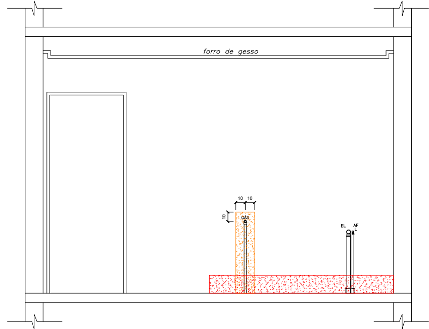
VISTA 1.0 - APARTAMENTO 602
