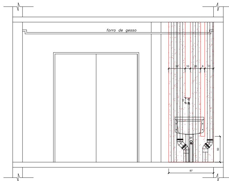
VISTA 2.0 - APARTAMENTO 610
