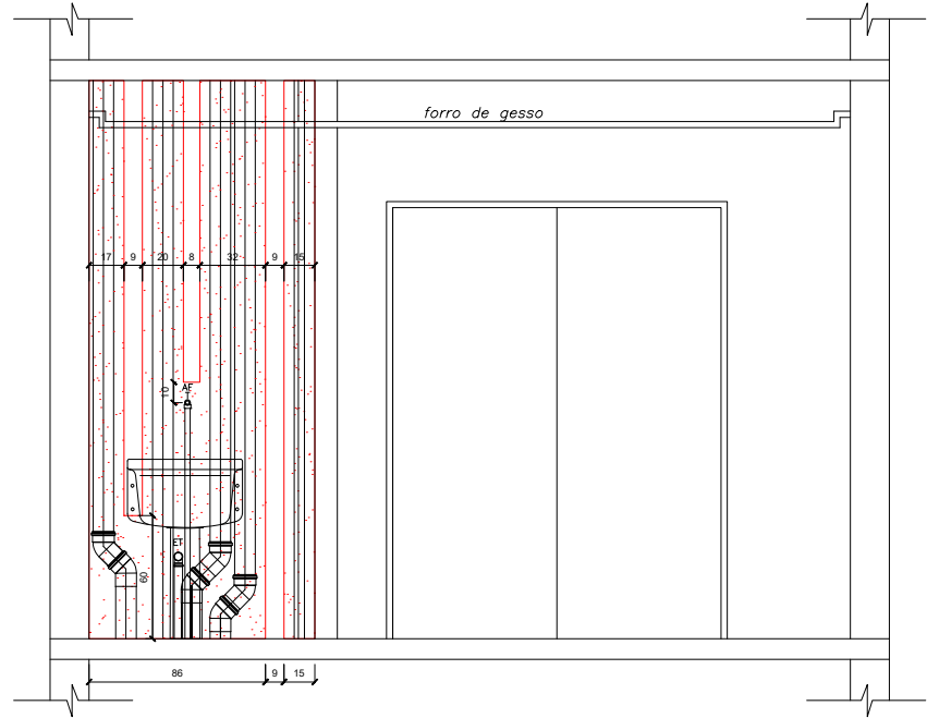
VISTA 2.0 - APARTAMENTO 608
