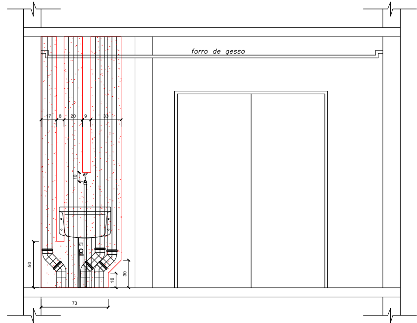
VISTA 2.0 - APARTAMENTO 613
