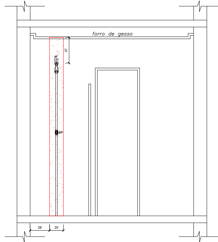
VISTA 3.0 - APARTAMENTO 608
