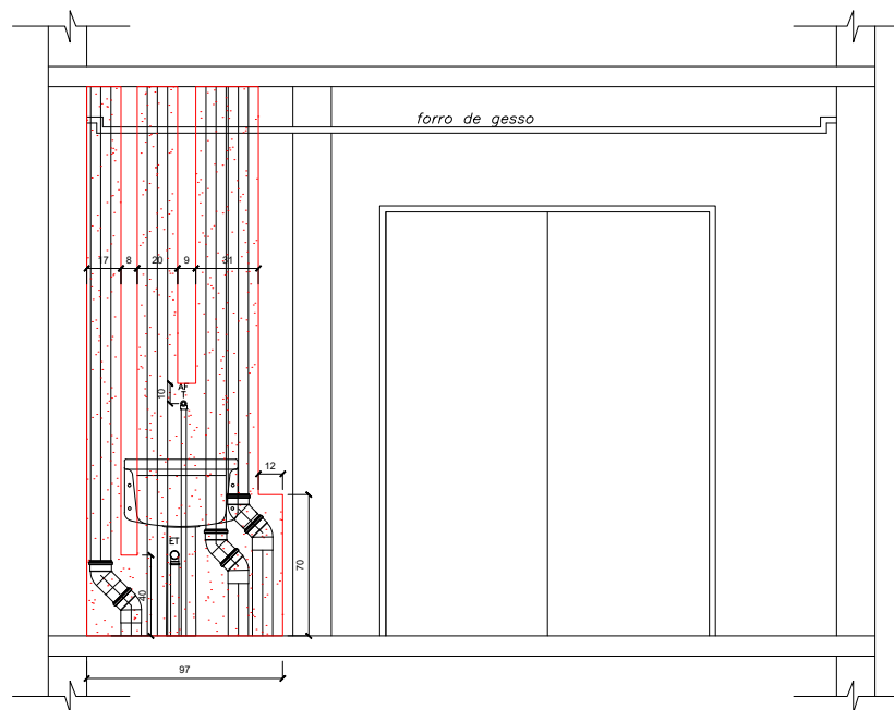
VISTA 2.0 - APARTAMENTO 612
