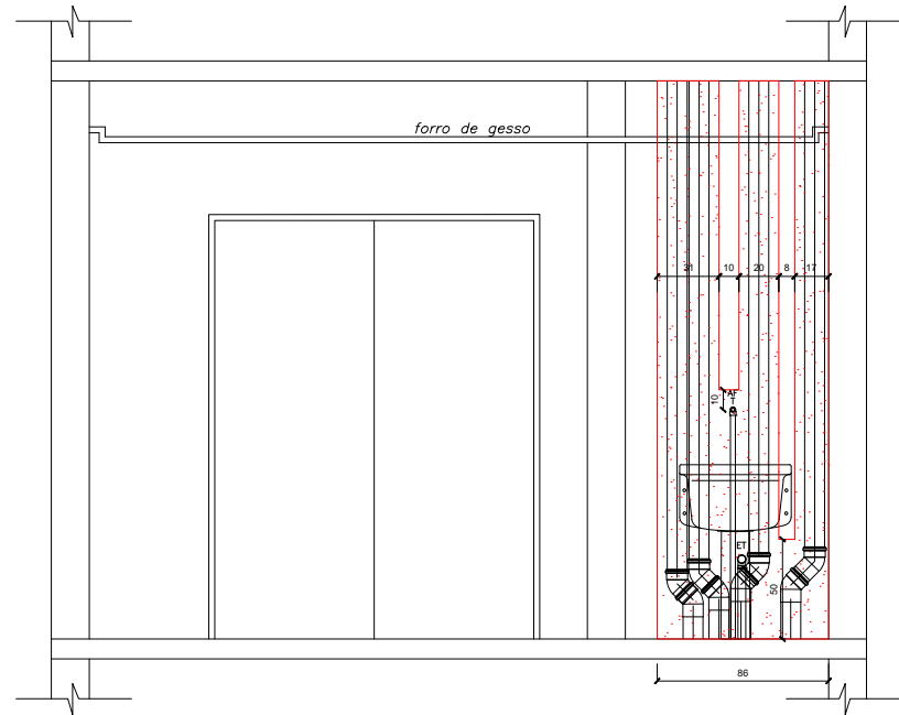
VISTA 2.0 - APARTAMENTO 614
