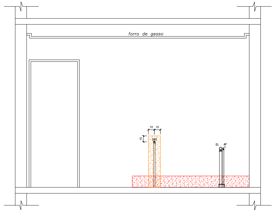
VISTA 1.0 - APARTAMENTO 704 A 1204
