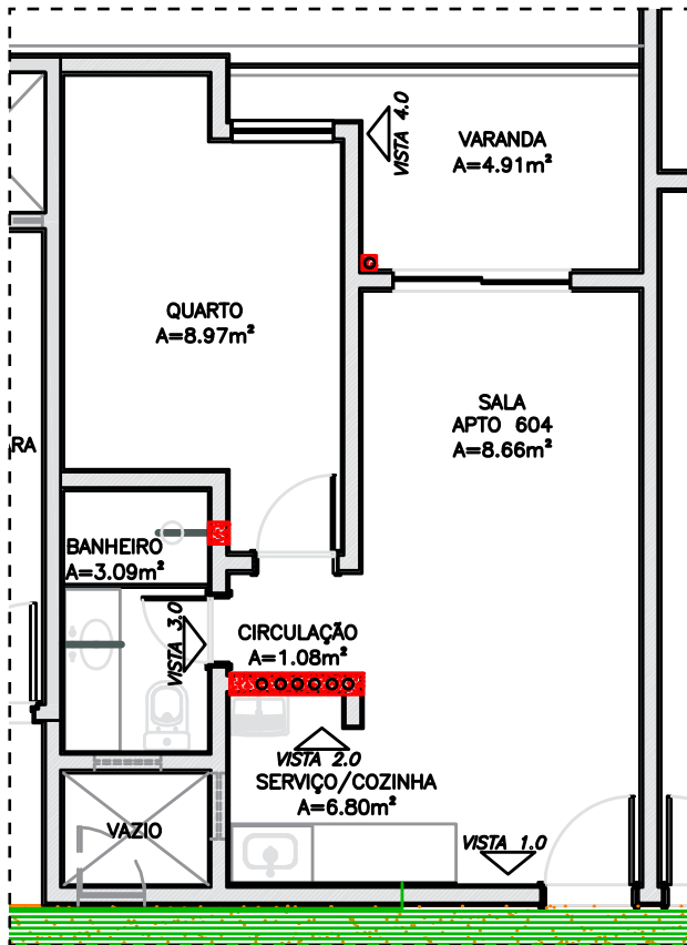
PLANTA APARTAMENTO 604
