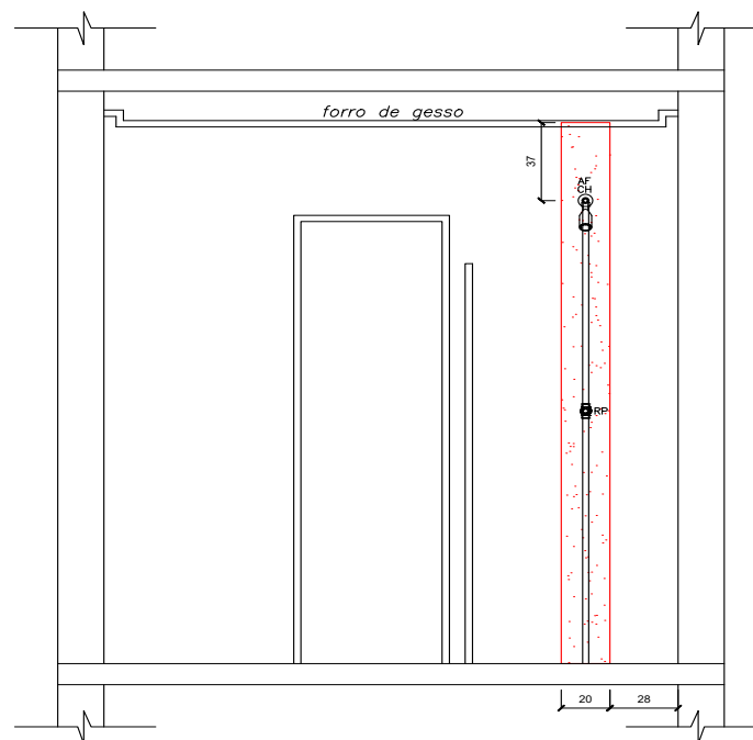
VISTA 3.0 - APARTAMENTO 615
