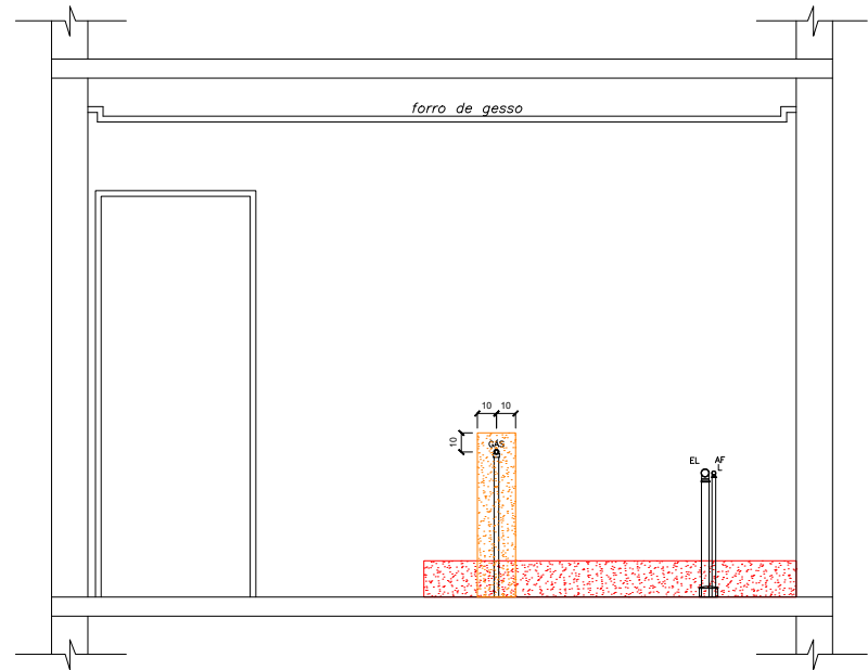
VISTA 1.0 - APARTAMENTO 702 A 1202
