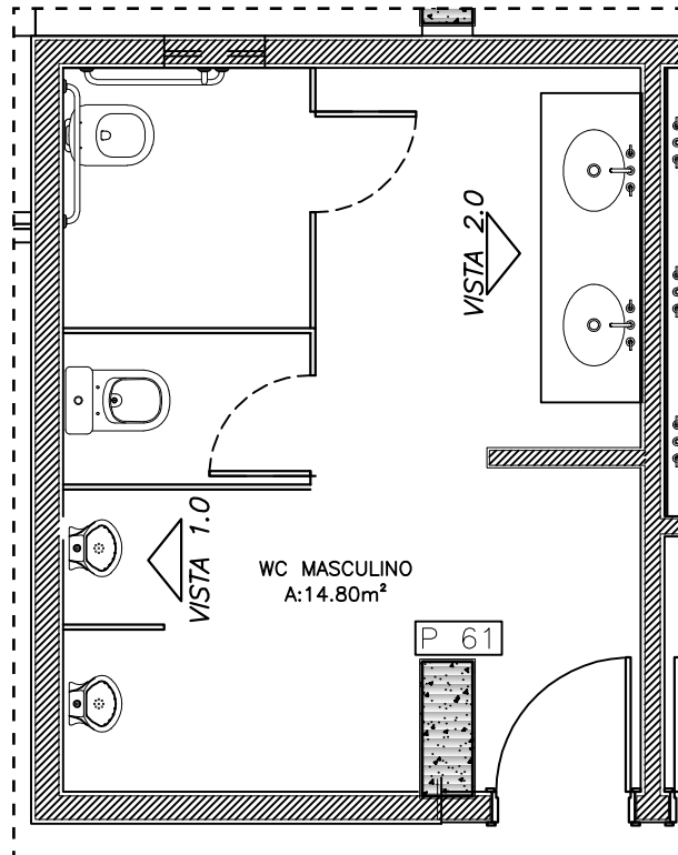
PLANTA WC MASCULINO
