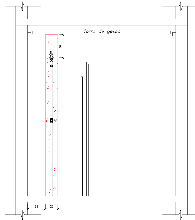
VISTA 3.0 - APARTAMENTO 602
