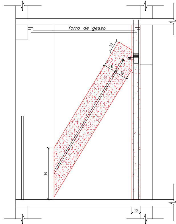
VISTA 4.0 - APARTAMENTO 607
