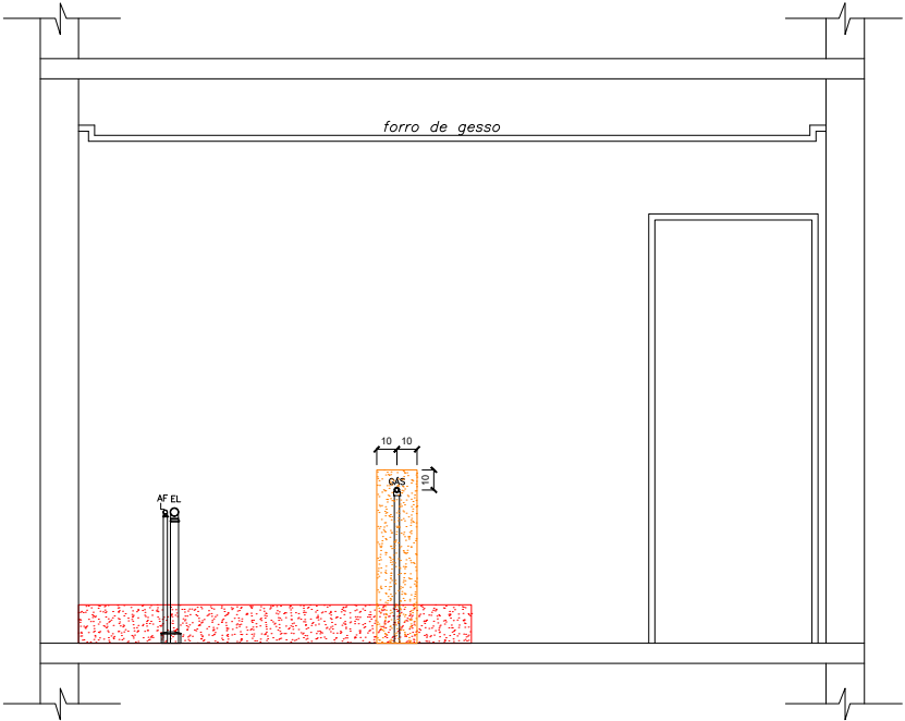
VISTA 1.0 - APARTAMENTO 614
