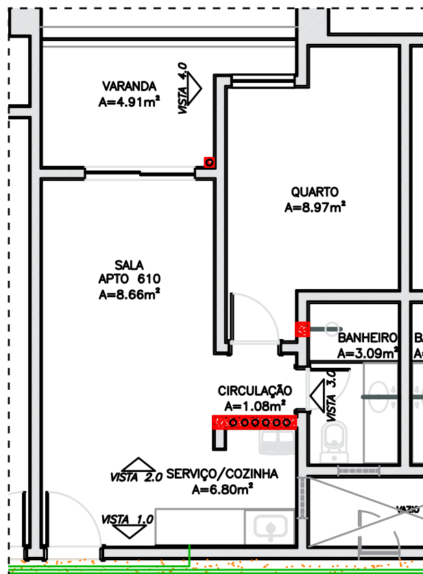
PLANTA APARTAMENTO 610
