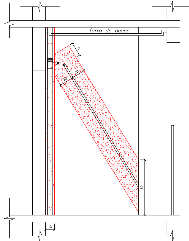
VISTA 4.0 - APARTAMENTO 613
