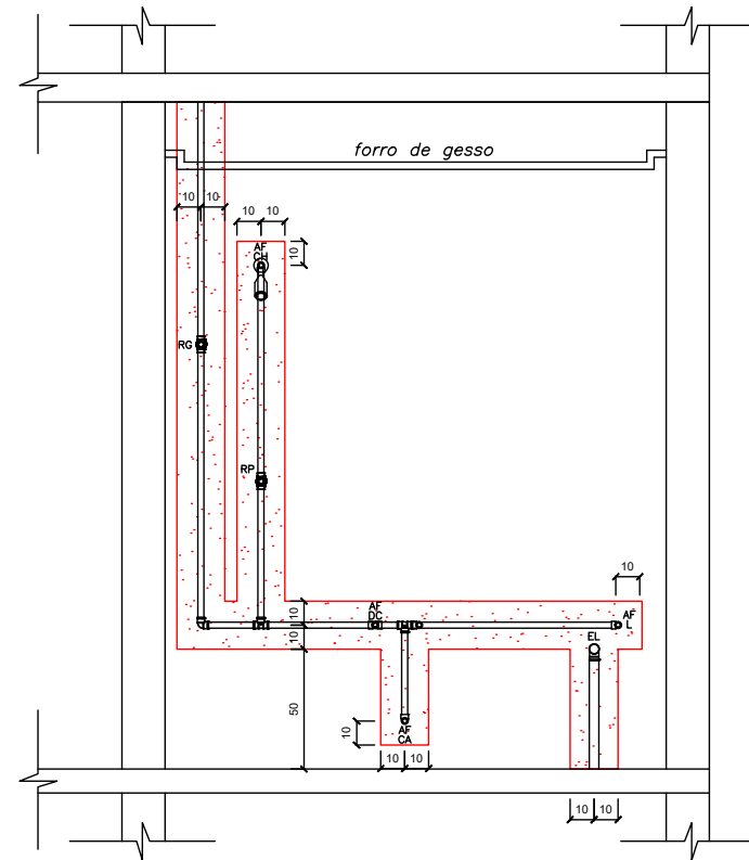
VISTA 1.0 - WC FUNCIONÁRIOS PORTARIA
