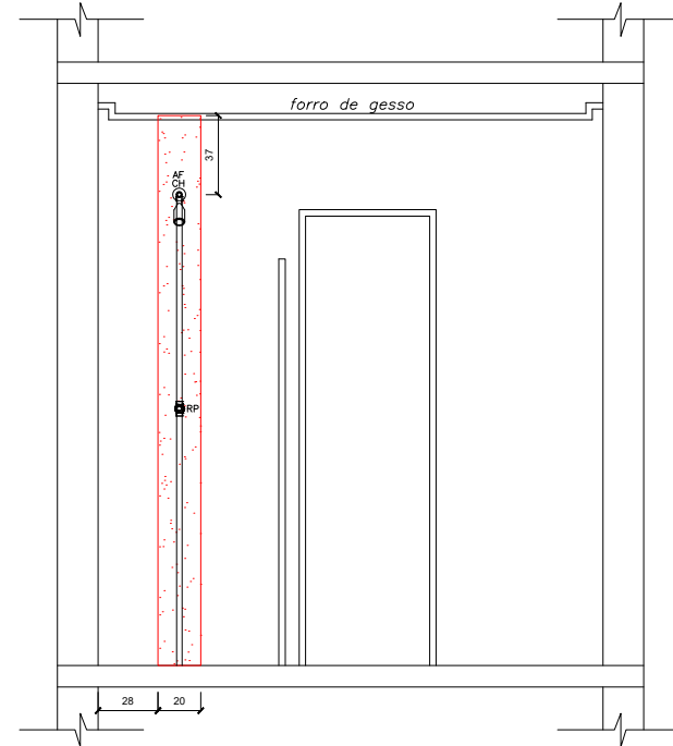
VISTA 3.0 - APARTAMENTO 601
