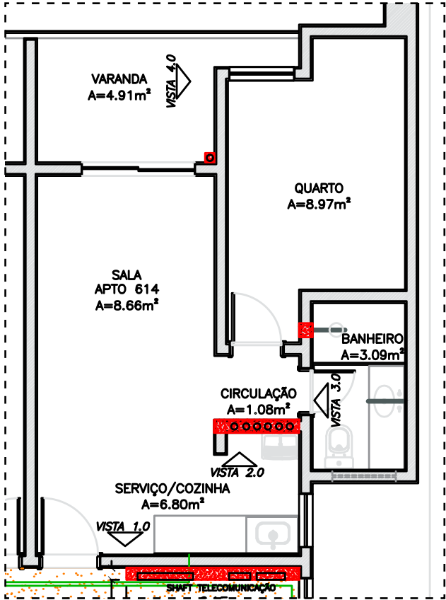
PLANTA APARTAMENTO 614
