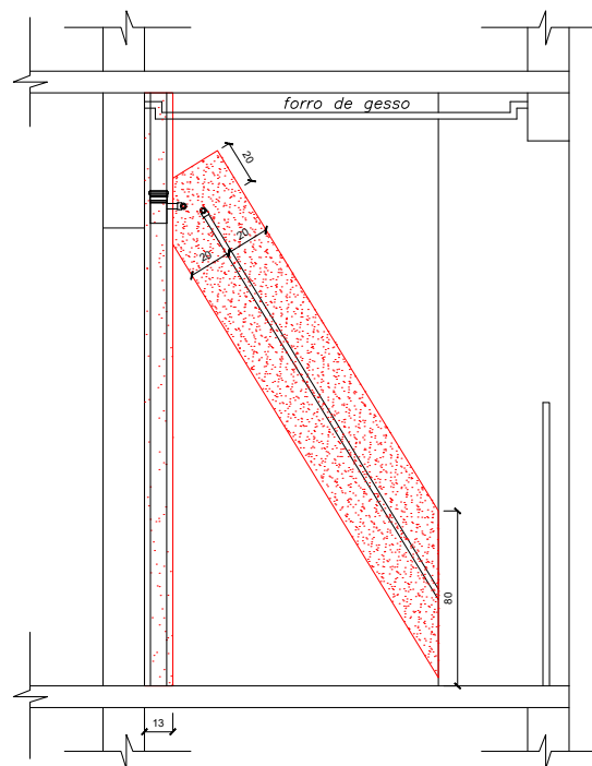
VISTA 4.0 - APARTAMENTO 602
