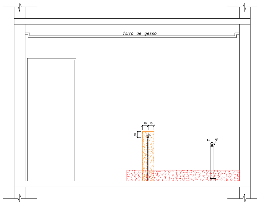
VISTA 1.0 - APARTAMENTO 604
