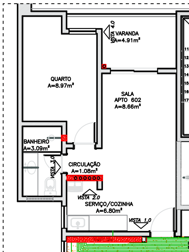
PLANTA APARTAMENTO 602
