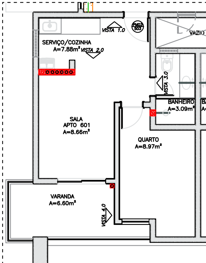
PLANTA APARTAMENTO 601
