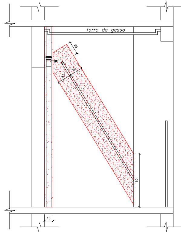
VISTA 4.0 - APARTAMENTO 702 A 1202
