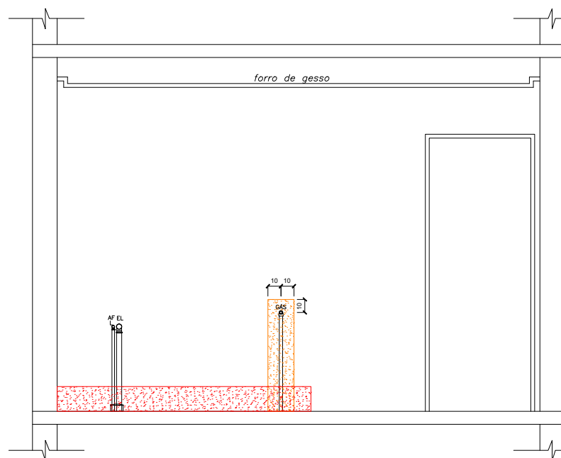
VISTA 1.0 - APARTAMENTO 601
