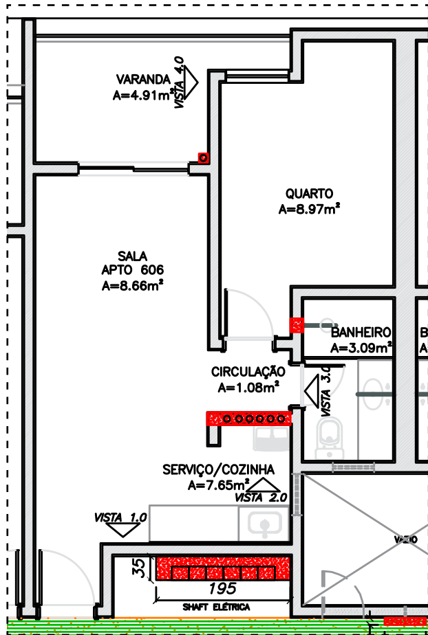
PLANTA APARTAMENTO 606
