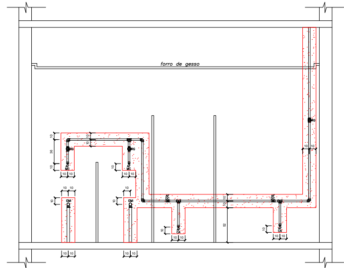
VISTA 1.0 - WC MASCULINO
