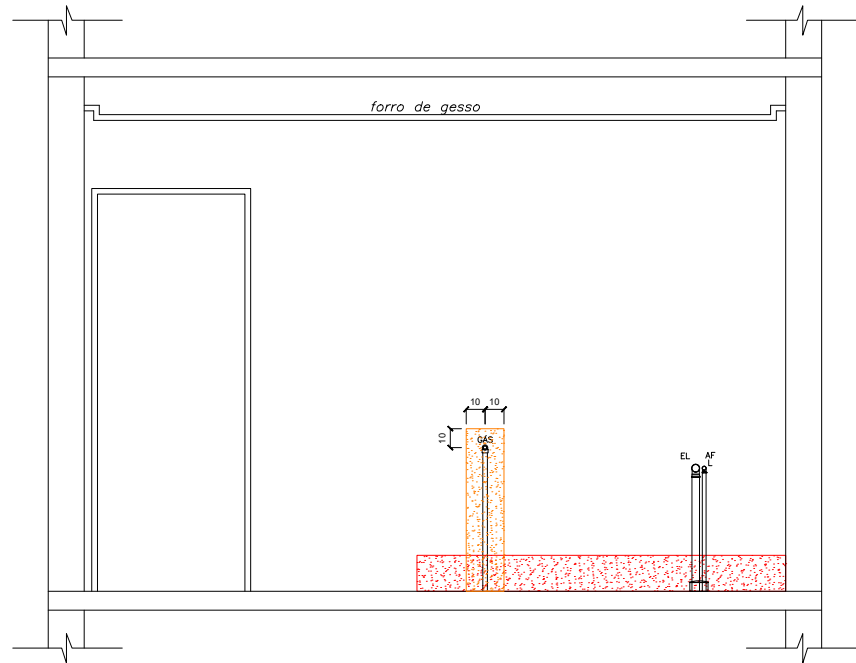
VISTA 1.0 - APARTAMENTO 613
