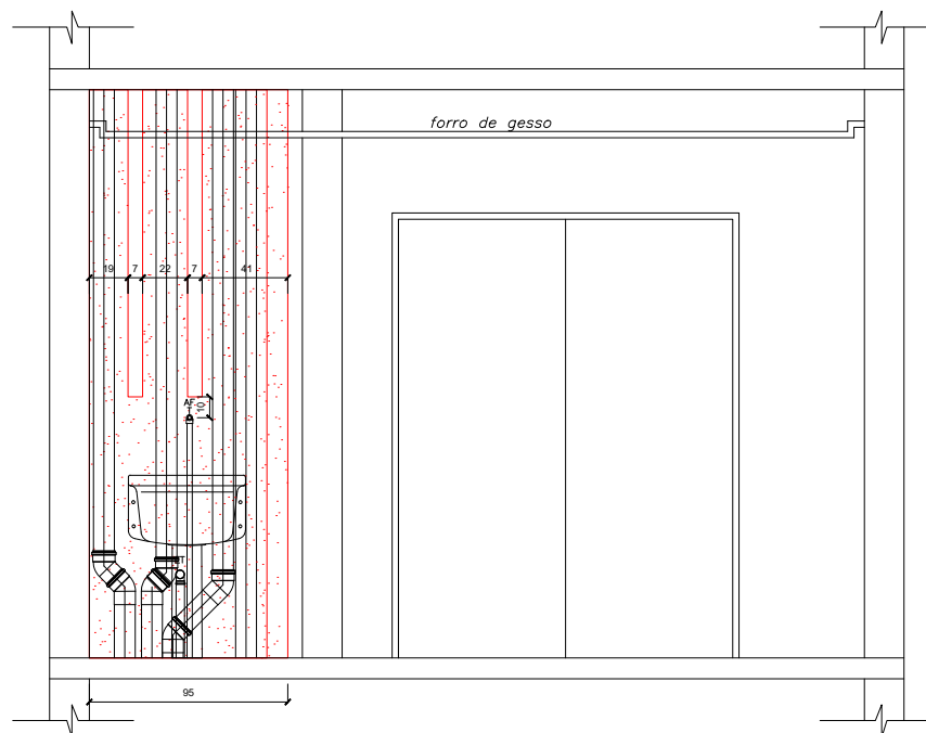
VISTA 2.0 - APARTAMENTO 605
