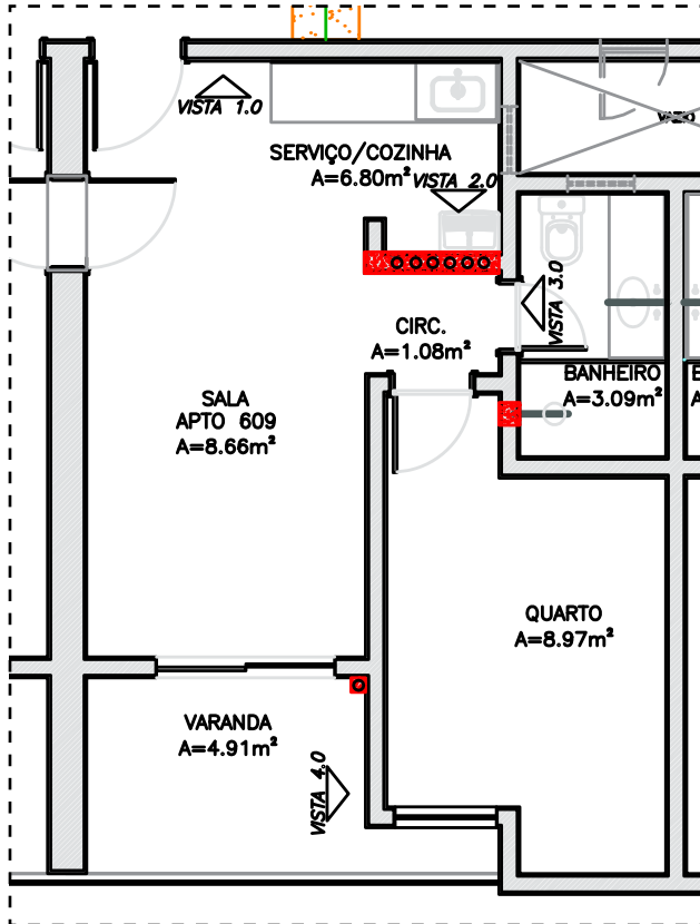
PLANTA APARTAMENTO 609
