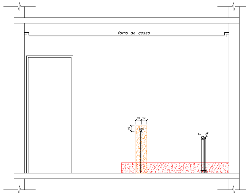
VISTA 1.0 - APARTAMENTO 615
