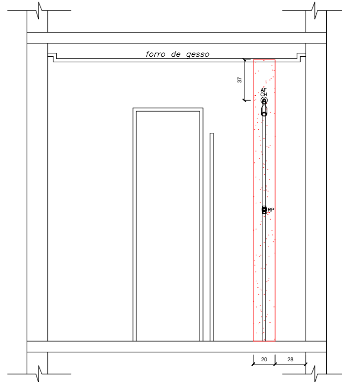
VISTA 3.0 - APARTAMENTO 603
