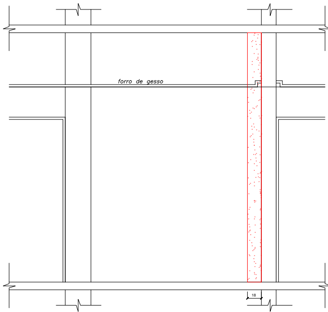
VISTA 1.0 - LAVANDERIA
