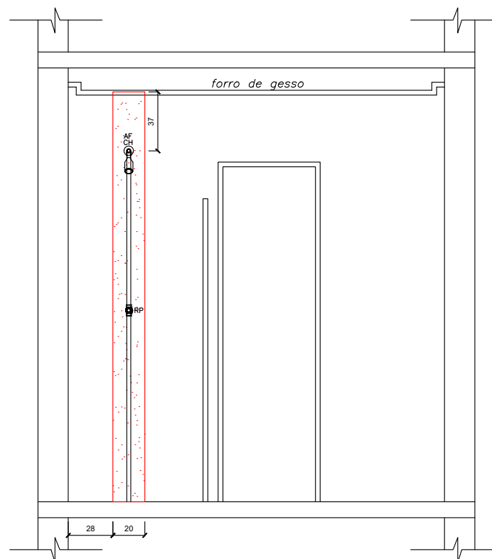
VISTA 3.0 - APARTAMENTO 613
