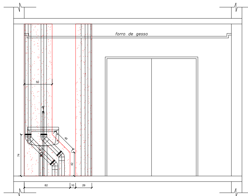
VISTA 2.0 - APARTAMENTO 615
