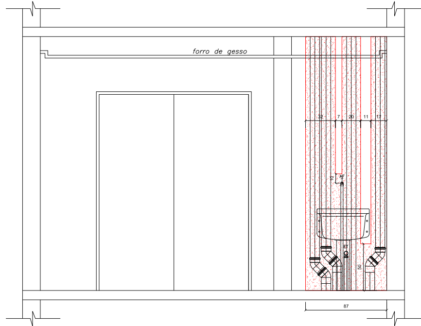
VISTA 2.0 - APARTAMENTO 606
