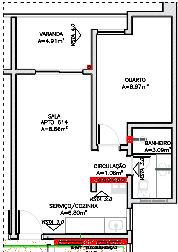
PLANTA APARTAMENTO 614
