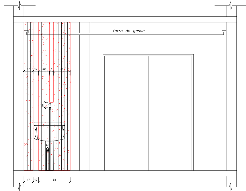
VISTA 2.0 - APARTAMENTO 704 A 1204
