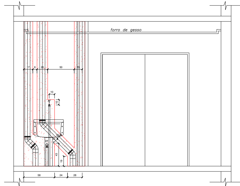
VISTA 2.0 - APARTAMENTO 609
