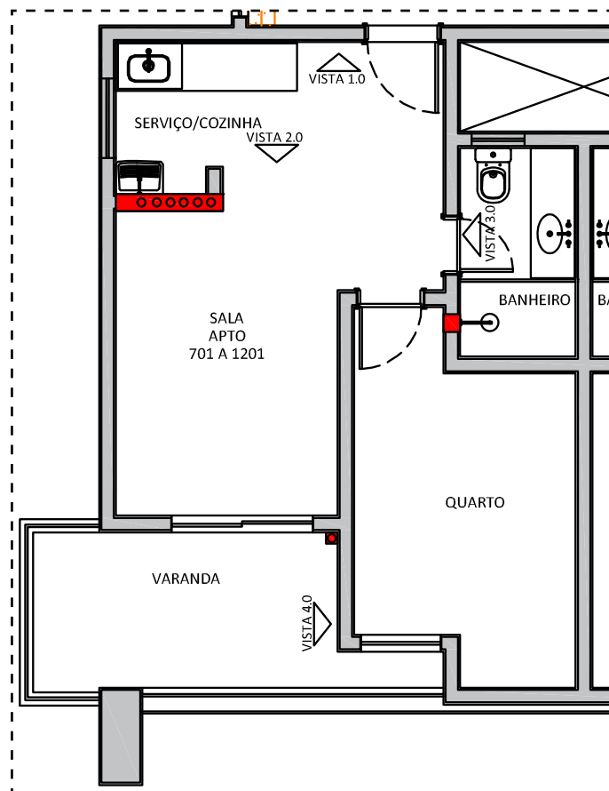
PLANTA APARTAMENTO 701 A 1201
