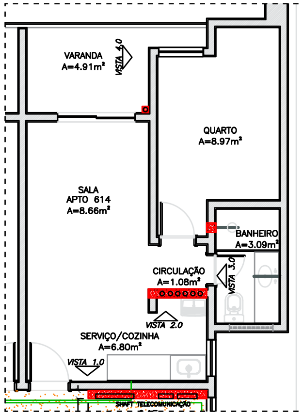
PLANTA APARTAMENTO 614
