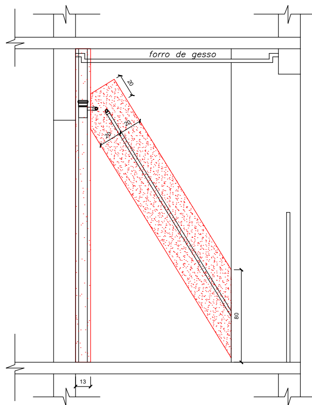
VISTA 4.0 - APARTAMENTO 605
