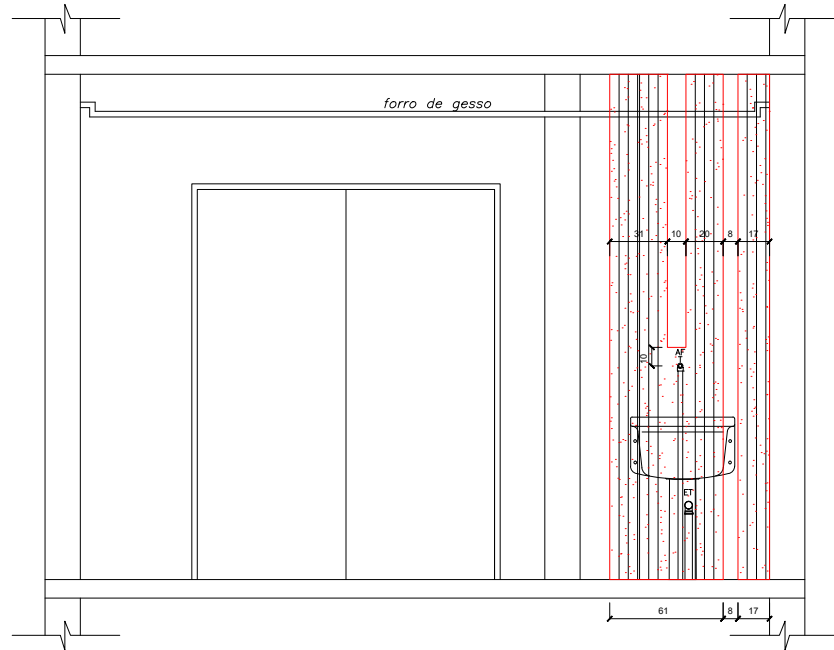
VISTA 2.0 - APARTAMENTO 703 A 1203
