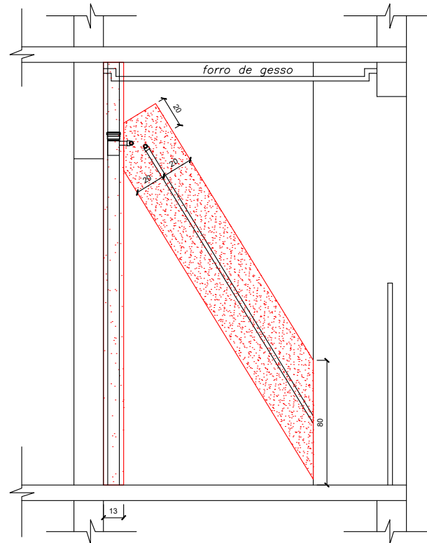
VISTA 4.0 - APARTAMENTO 608
