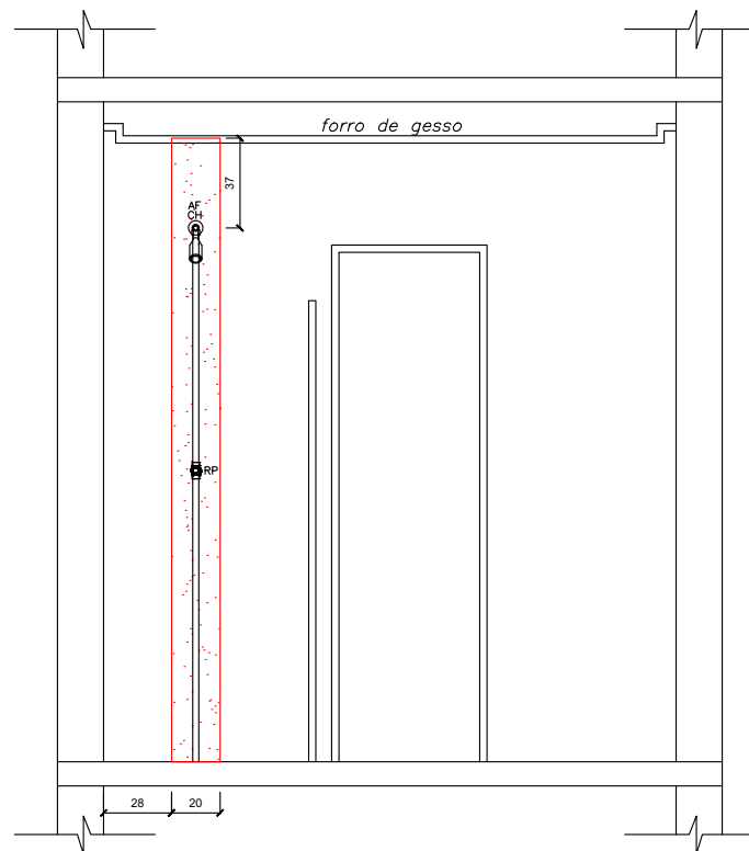
VISTA 3.0 - APARTAMENTO 604
