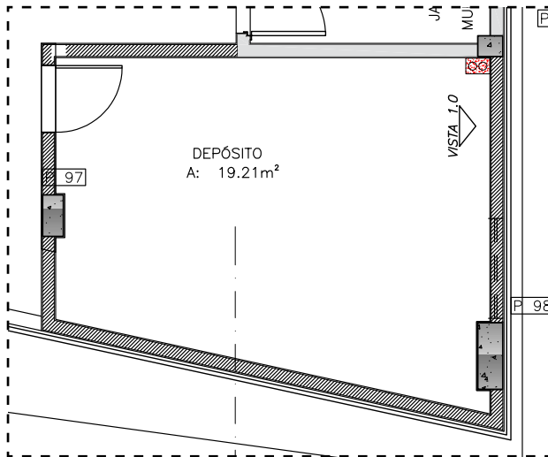
PLANTA DEPÓSITO
