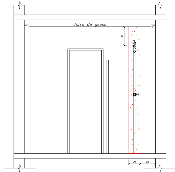
VISTA 3.0 - APARTAMENTO 607
