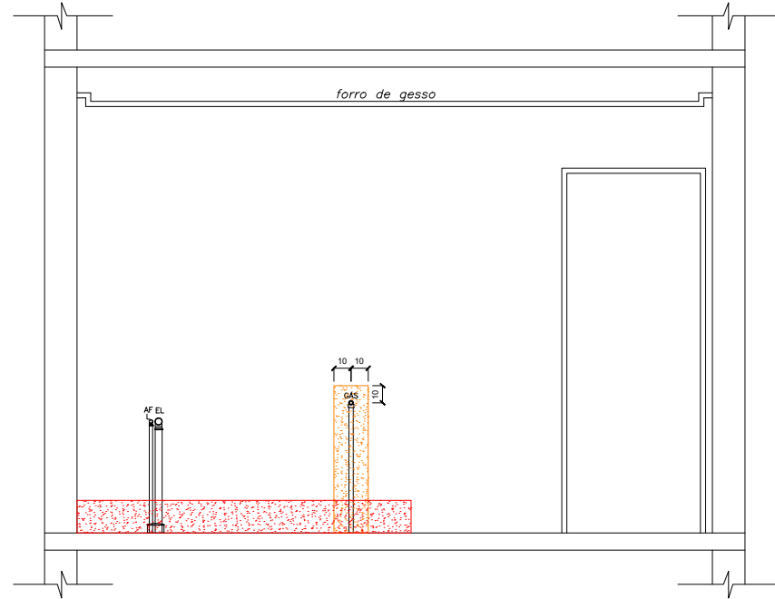
VISTA 1.0 - APARTAMENTO 610
