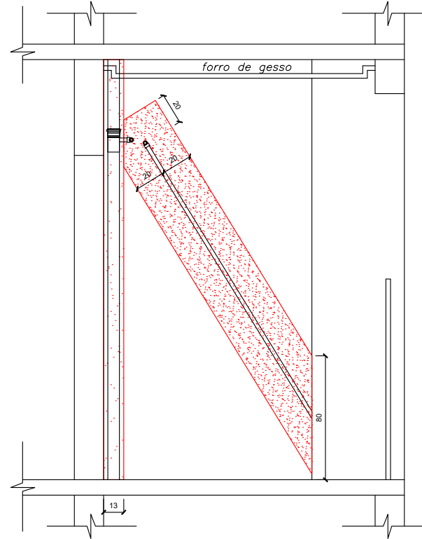
VISTA 4.0 - APARTAMENTO 609
