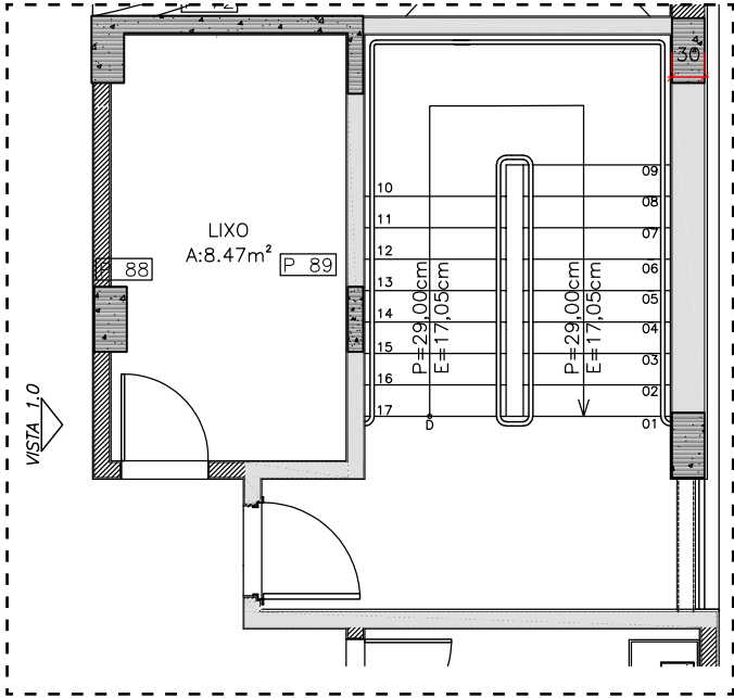
PLANTA LIXO
