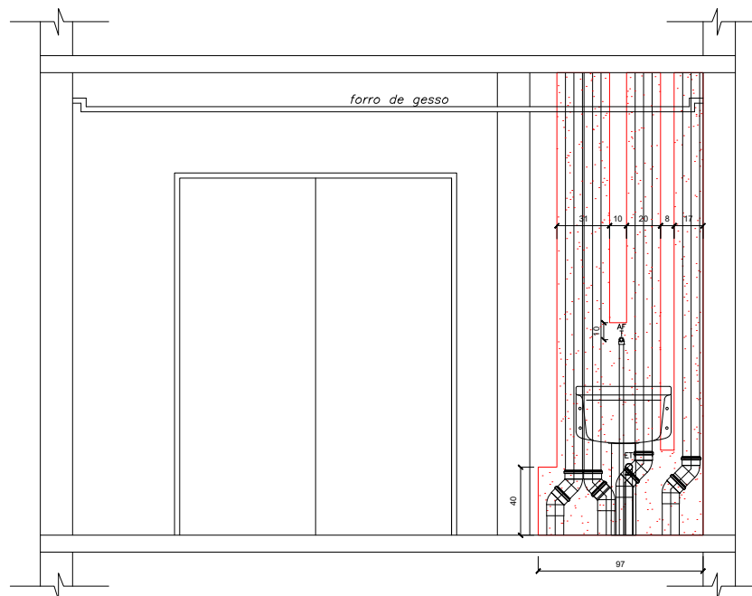
VISTA 2.0 - APARTAMENTO 607
