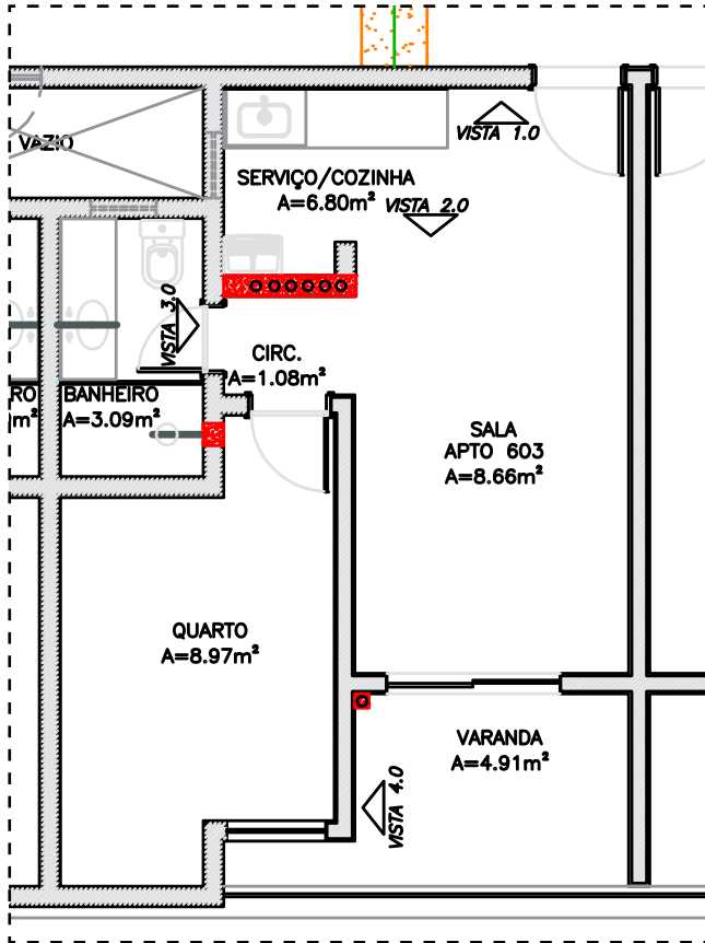
PLANTA APARTAMENTO 603
