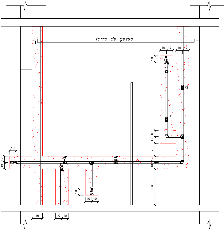
VISTA 1.0 - WC SERVIÇO
