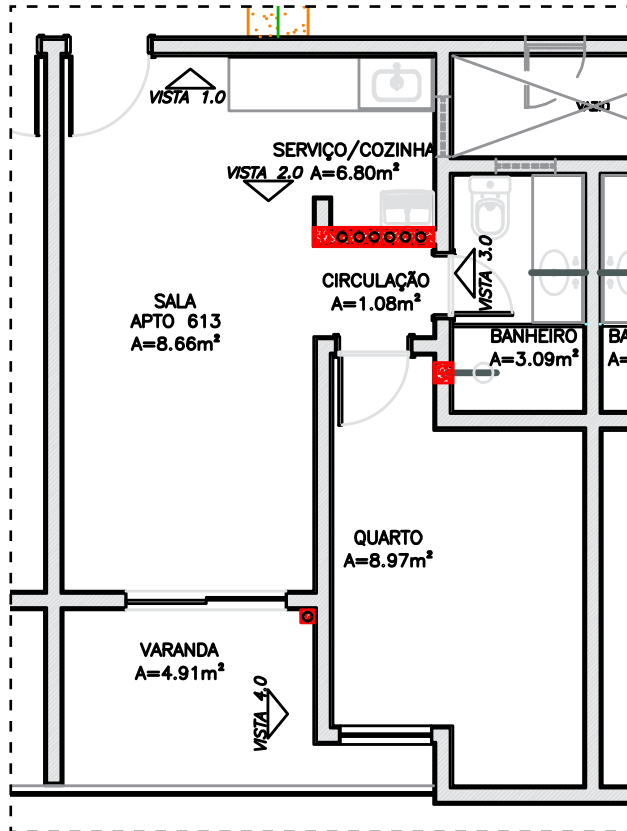
PLANTA APARTAMENTO 613
